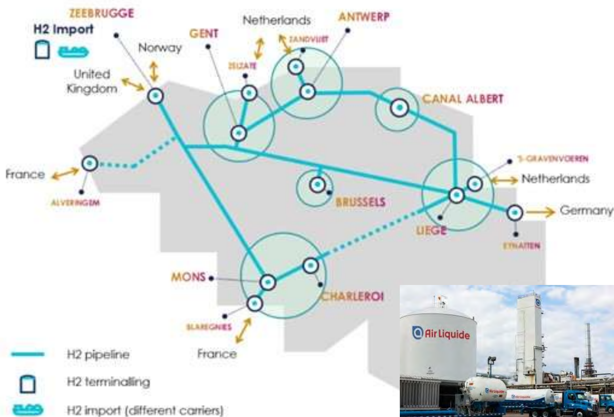
Overzicht van de waterstofleidingen in België.
